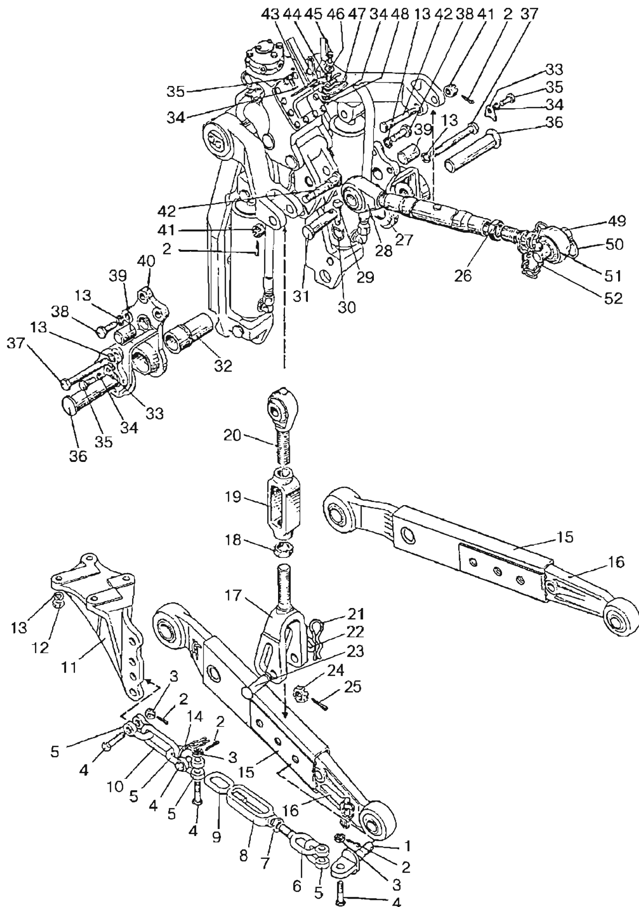
Рис. 46.2. Механизм задней навески (вариант для трактора «БЕЛАРУС-82П» с гидрорподъемником)
