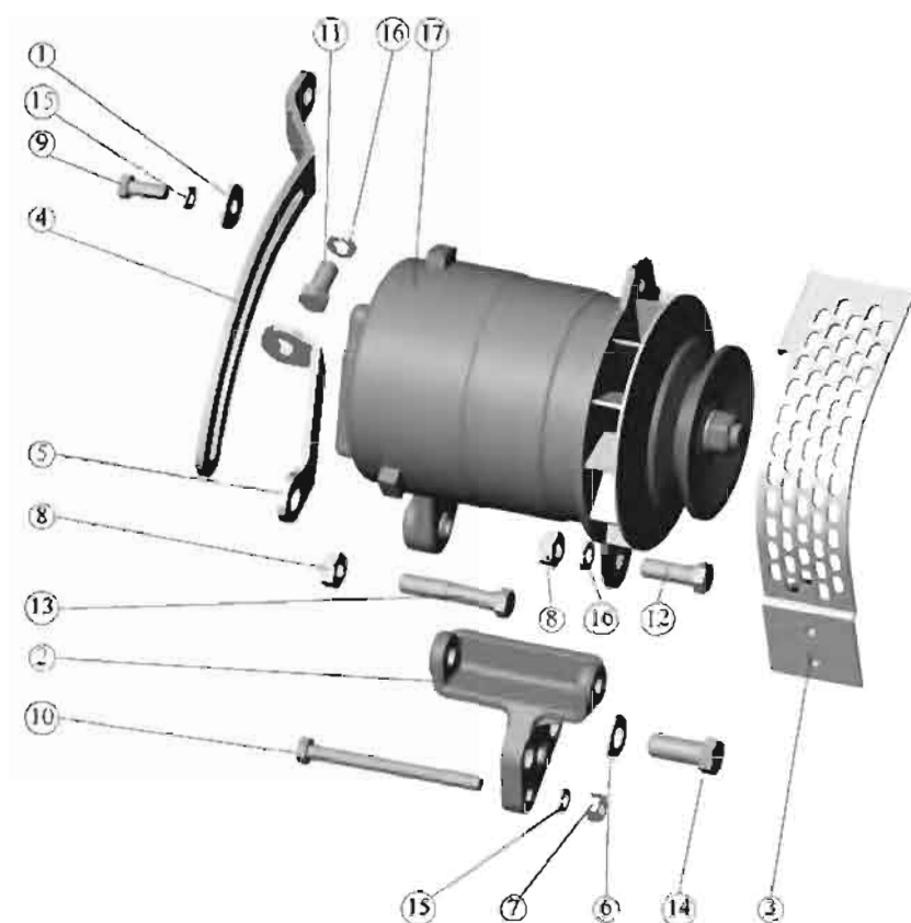
Рис. 37.7. Генератор (для трактора «БЕЛАРУС-80.1/80.Y/82Y/82.1/820/82P/82П»)
